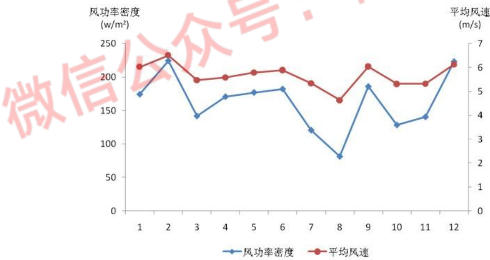
图4-2 各月平均风功率密度和平均风速变化曲线
